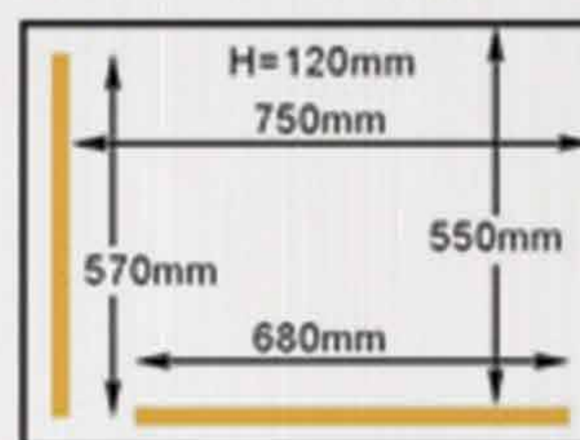
DZ-800/2L
